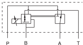
型号 3DREP-02B
