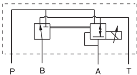
型号 3DREP-02A
